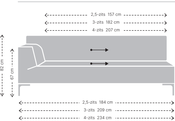
HOOGTE X BREEDTE
