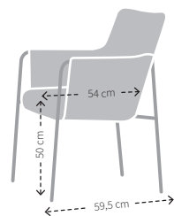
DIEPTE, ZITDIEPTE EN ZITHOOGTE
